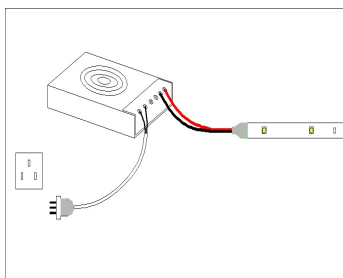
将 LED 灯带连接到 LED 驱动器输出侧 (正极接正极，负极接负极。)
