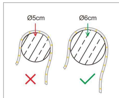
弯曲灯带曲面直径不可小于 6cm
