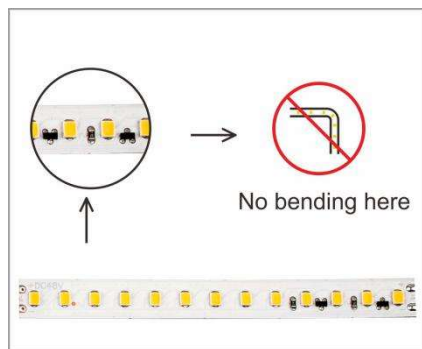
禁止在灯珠处弯曲灯带
