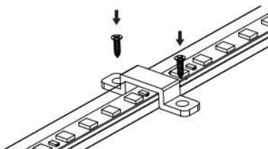
将灯带固定在安装表面，使用卡子固定
